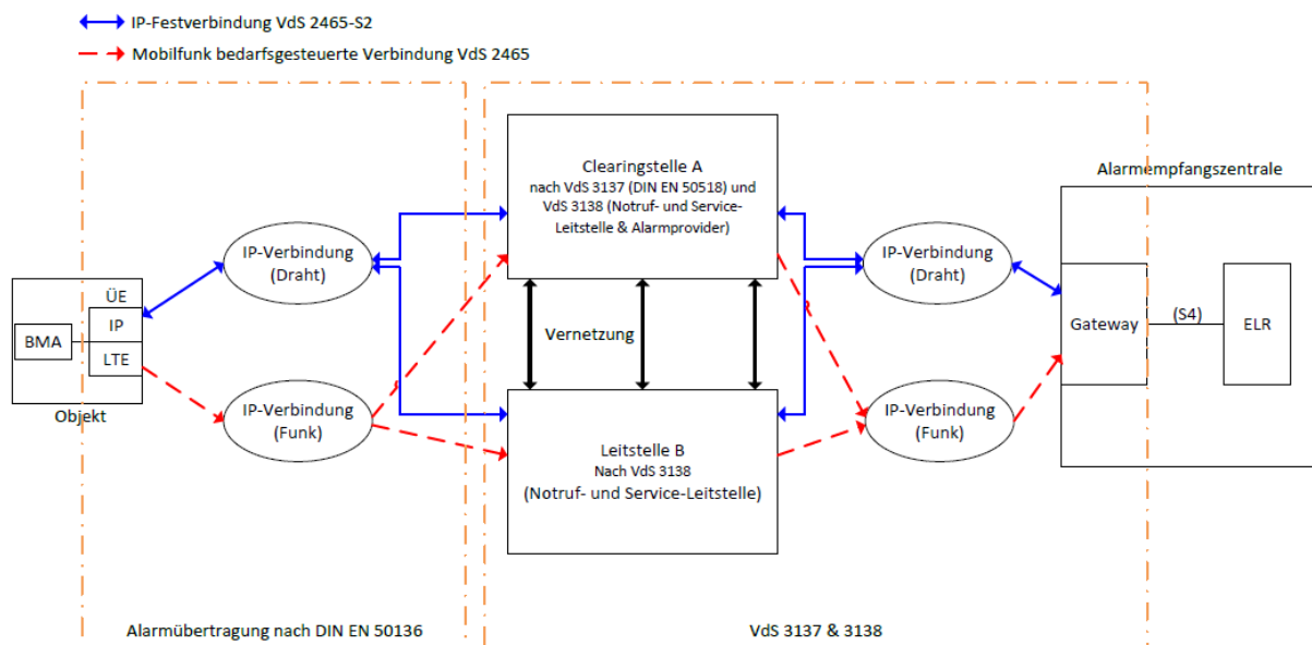
Abbildung 1: Systemübersicht AÜA
